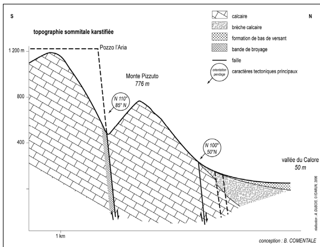
Figure 2 - Coupe le long de la bordure nord du Camposauro.
