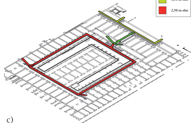
Fig. 22 – Ostie. Évolution du schéma de circulation dans les Grandi Horrea : a) à la fin du II e siècle b) lors de la première phase sévérienne c) lors de la seconde phase sévérienne (DAO N.M.).
