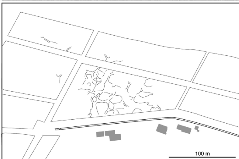
Figure 4 : Grands polygones en vue aérienne apparaissant dans la parcelle au sud du Lac Bleu en période de stress hydriques des plans de vigne. Gauche : vue Google Earth du 31/08/2006 ; droite : dessin des linéations observables sur cette même vue.
