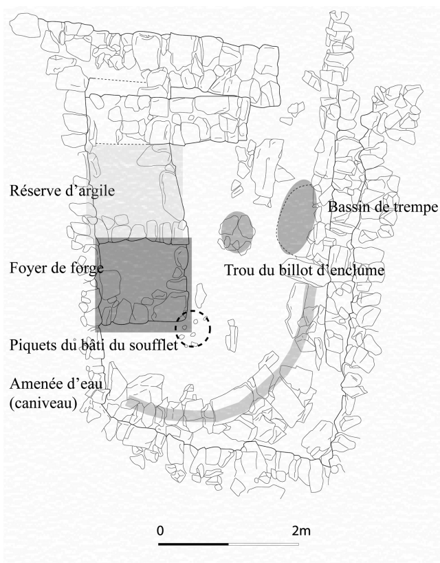
Figure 6 : Plan type des forges de Brandes.
