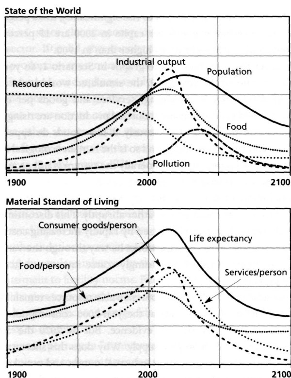
Un des scénarios de Meadows et al. 2008
