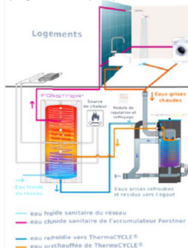
Figure 3. Association du ThermoCycle®WRG avec un ballon accumulateur à stratification de la gamme FORSTNER (source énergie efficiente)
