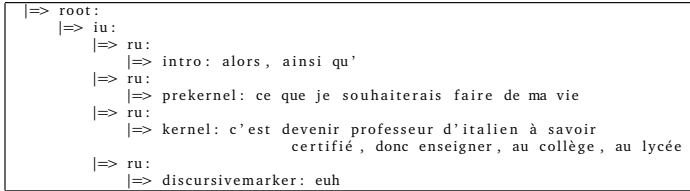
FIGURE 10 – Arbre projeté de macro-syntaxe résultant de l'analyse de a .
