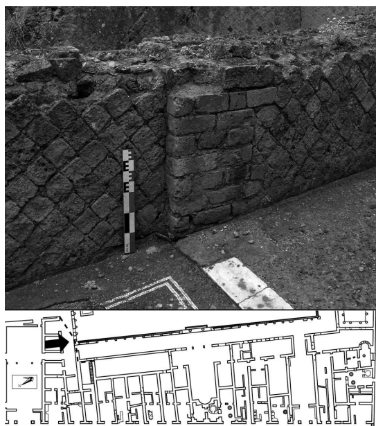
Fig. 9. Pièce 19-3 de la loggia, mur sud. La césure verticale visible dans la maçonnerie originelle montre que les niveaux de circulation situés au-dessus de l'extrados du cryptoportique se s'appuient sur les constructions constituant l'angle nord-ouest de l'édifice.
