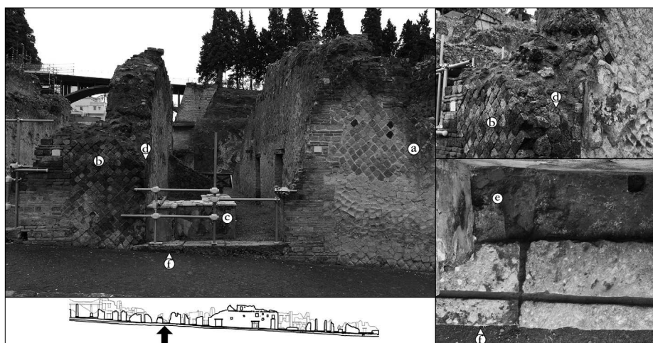
Figure 19. Entrée du commerce alimentaire Or. II, 13. La construction originelle (a) se distingue des réparations effectuées sous Vespasien (b). Pour installer un comptoir (c), le montant reconstruit a été taillé (d) et partiellement arasé. Ses vestiges apparaissent (e) sous la pierre de seuil alors ajoutée (f).
