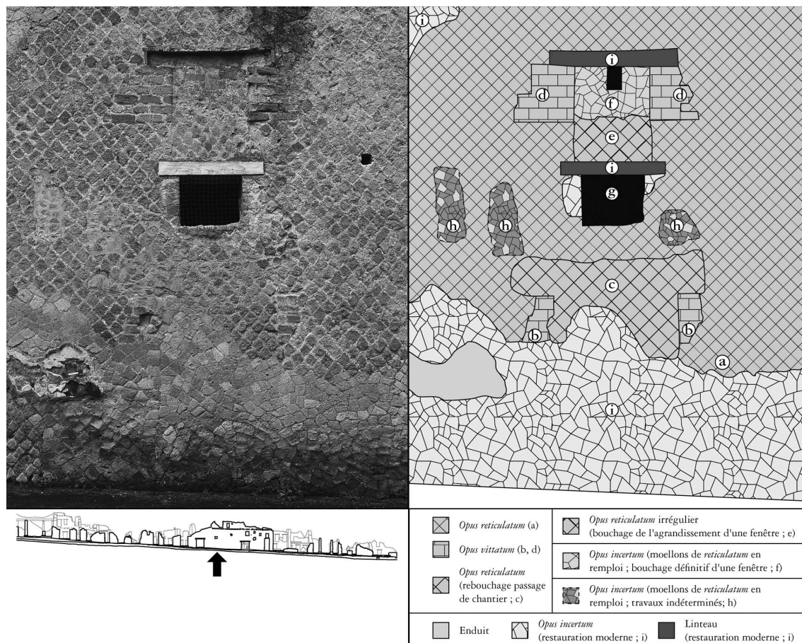
Fig. 7. Façade extérieure de la pièce 8-5. L'observation des différents types de maçonnerie permet de restituer des phases distinctes. Lors de la construction originelle (a), un passage de chantier est ménagé : deux montants (b) permettent l'insertion temporaire d'un linteau, enlevé à la fin des travaux. Le passage est alors rebouché (c). Une fenêtre est prévue dès l'origine (d). Lors de l'usage du bâtiment, elle est agrandie puis partiellement rebouchée (e). Elle est définitivement condamnée lors des travaux de Vespasien (f), ce qui n'empêche pas sa réouverture dans un second temps (g). La paroi présente des réparations (h) qu'il est impossible en l'état d'assigner à une phase particulière, mais qui sont distinctes des restaurations modernes (i).
