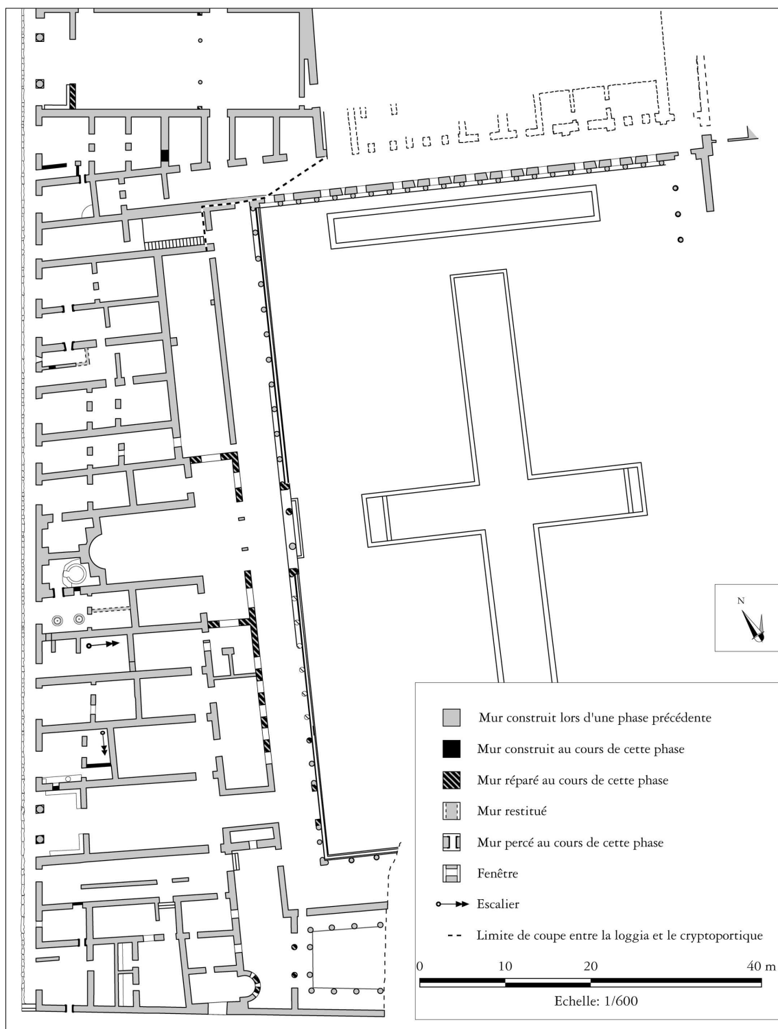
Fig. 16. Restitution du plan de la seconde phase de l' Insula Orientalis II a entre le séisme de 62 et celui du début des années 70 (DAO N. Monteix, d'après relevé F. Ferrajoli modifié par L. Trinca et M.R. Acetoso).
