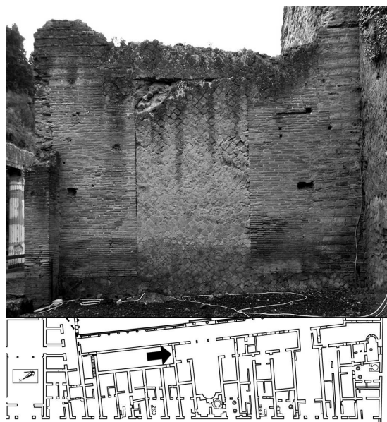
Fig. 14. Mur de séparation entre le pronaos et la salle L (cliché N. Monteix).
