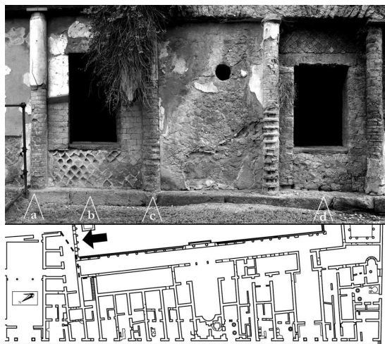
Fig. 8. Partie ouest du cryptoportique donnant sur la terrasse inférieure. D'abord construites en opus vittatum (a), les colonnes s'appuient sur un massif en opus reticulatum continu à la base des fenêtres (b). Elles sont ensuite construites en opus vittatum mixtum à une assise de briques (c), alors que la base des fenêtres n'est plus construite de façon continue, mais dans un second temps du chantier (d).
