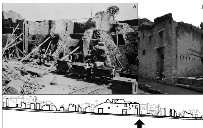
Fig. 4. Deux états de la façade. A. lors de son dégagement en 1932 ; on note les échafaudages et la maçonnerie à peine refaite (cliché SANP, E/C 217, 1932). B. en 2008 ; la distinction entre la maçonnerie antique et celle de restauration est parfois délicate.
