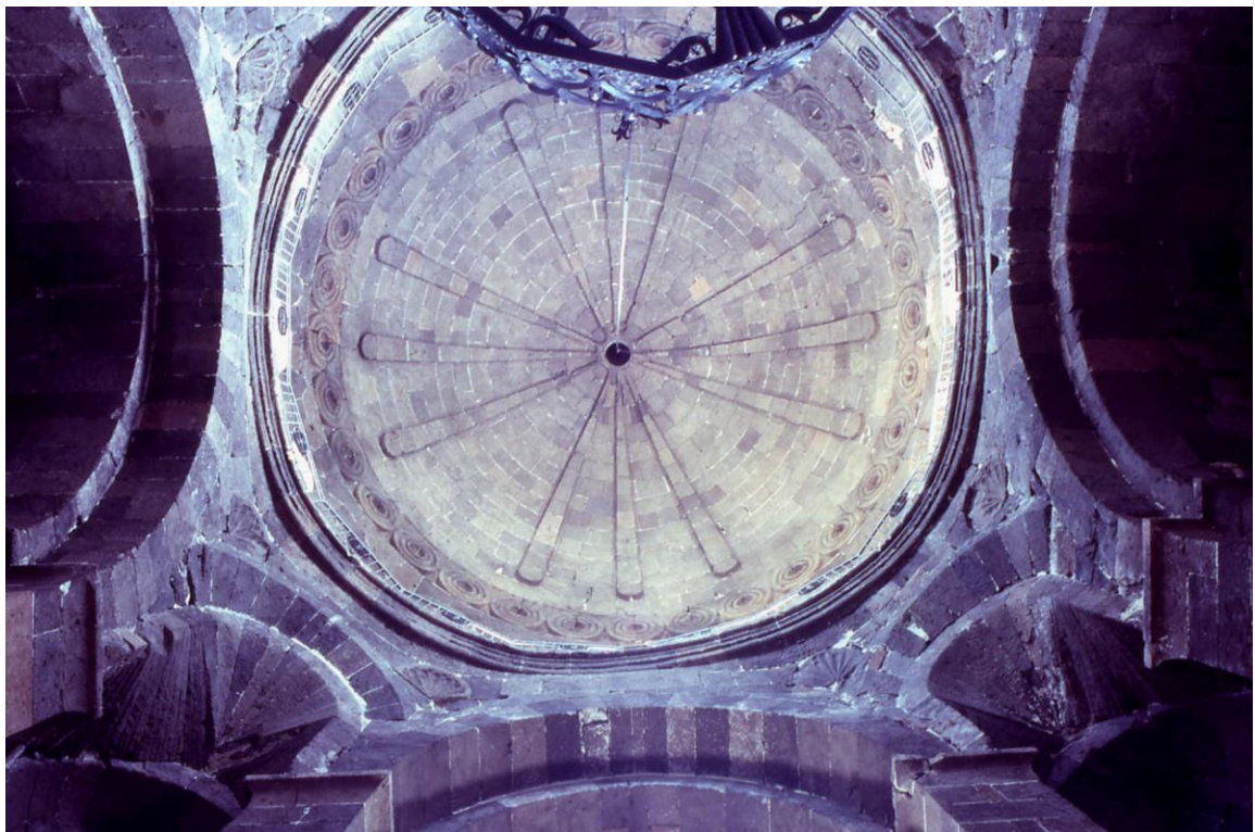
Fig. 22. Vałaršapat, ęglise Sainte-Rhipsimę, coupole, trompes et trompillons.
