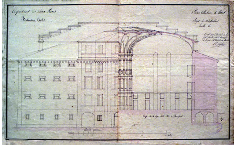
Fig. 18- Coupe sur la grande voûte annulaire, dessin de P. Th. Segretain (AD79, 4N54, © Chantal Callais)
