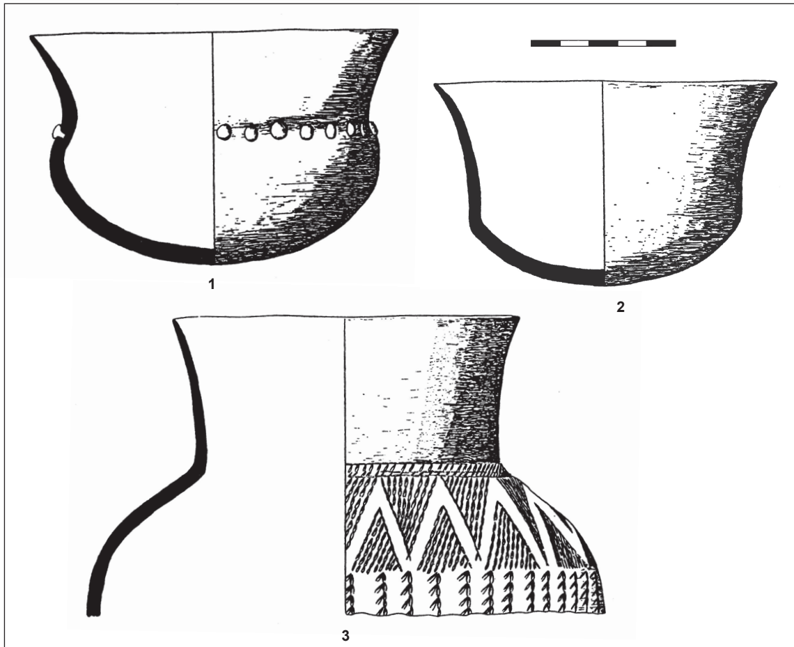
Fig. 8. Entzheim « Sablière Oesch ». Mobilier céramique de la fosse 1. Phase 1 du BORS (d'après SCHMITT, 1974).
