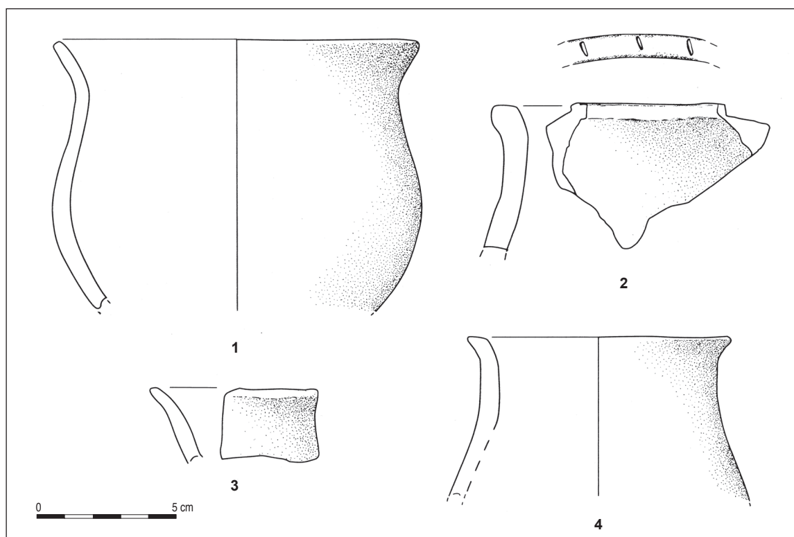
Fig. 4. Rosheim « Rittergass ». Céramiques grossières de la fosse 2020 (éch. 1:2; dessin P. Lefranc/A. Serrurier).
