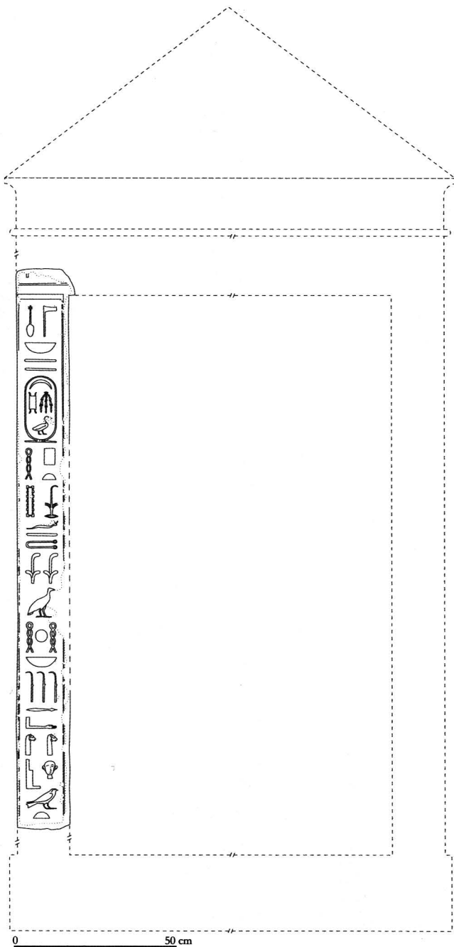
Pl. 2. Proposition de restitution du naos d'Amasis (© Cnrs-Cfeetk/Chr. Thiers).
