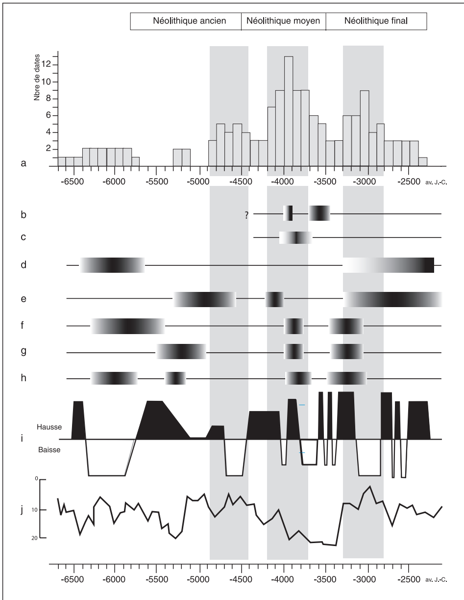
Fig. 4 - Comparaison entre les rythmes d'anthropisation enregistrés sur les Pyrénées à partir des indices polliniques d'anthropisation et les variations du climat européen, entre -6500 et -2500 mise en évidence par plusieurs archives climatiques : (a) distribution chronologique des dates d'apparition des indices polliniques d'anthropisation ; (b) avancées glaciaires enregistrées dans le cirque de Troumouse (Pyrénées centrales) (Gellatly et al. 1992) ; (c) phase de haut niveau lacustre enregistrée dans les Pyrénées-orientales (Guiter et al. 2005) ; (d) phases d'aridification du climat du bassin nord-occidental de la Méditerranée (Jalut et al. 2000) ; (e) phases de réduction des glaciers dans les Alpes suisses (Hornes et al. 2001) ; (f) avancées glaciaires dans les Alpes suisses (Zoller 1977) ; (g) avancées glaciaires dans les Alpes autrichiennes (Patzel 1977 in Haas et al. 1998) ; (h) phases froides et humides en Europe (Haas et al. 1998) ; (i) variations des niveaux lacustres dans le Jura (Magny 1999) ; (j) variations des lithoclastes dans les sédiments marins en Atlantique-Nord ( Ice-Rafted Debris ) (Bond et al. 2001 in Heiri et al. 2004).
