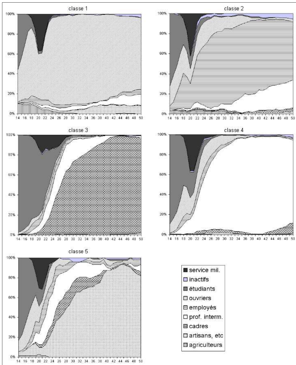
Figure 5 – Chronogrammes de la typologie en cinq classes 35
