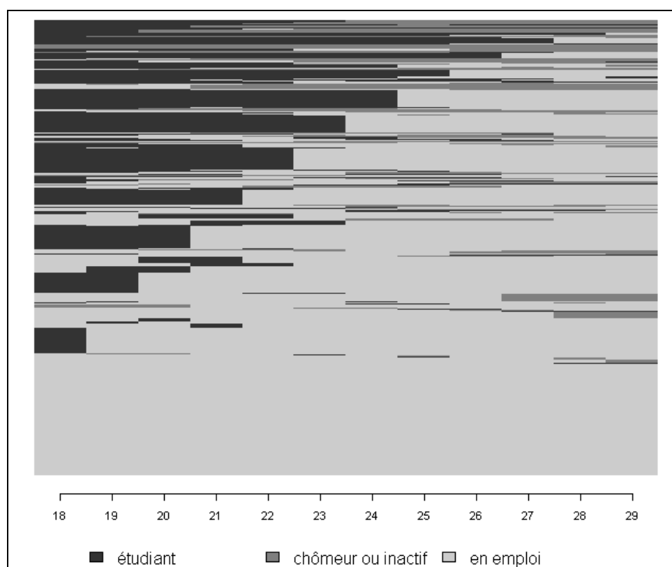
Figure 3 – Tapis de trajectoires d'insertion
