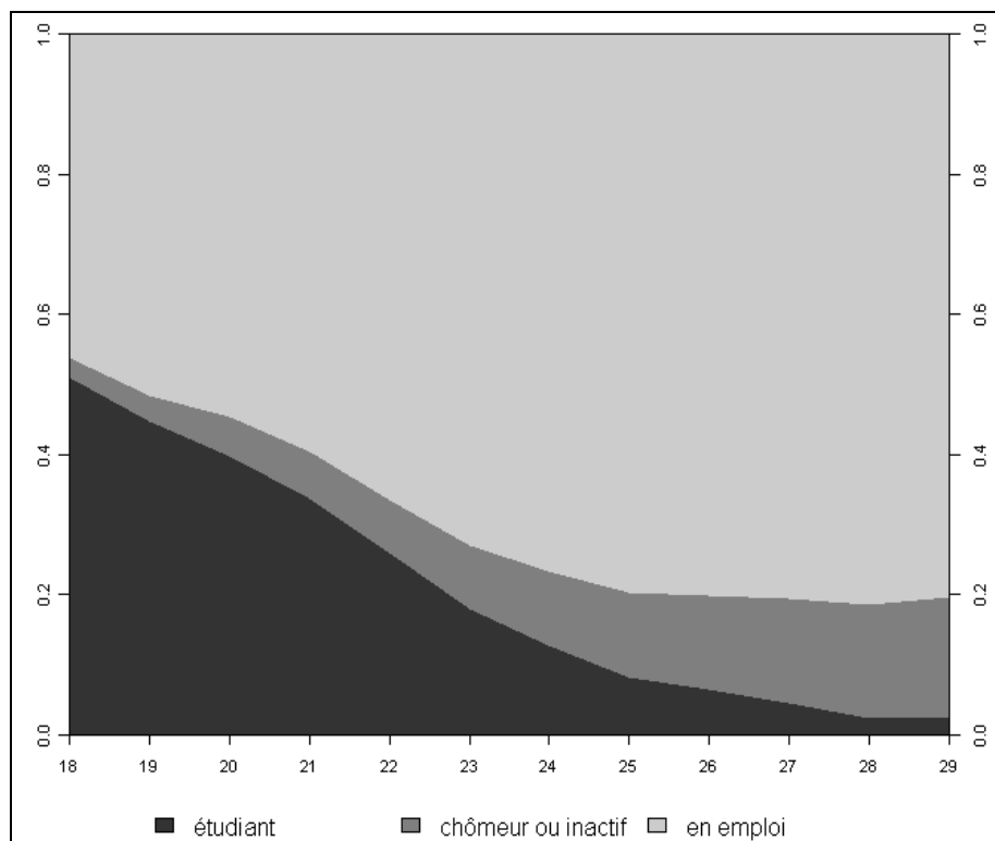
Figure 2 – Chronogramme de trajectoires d'insertion
