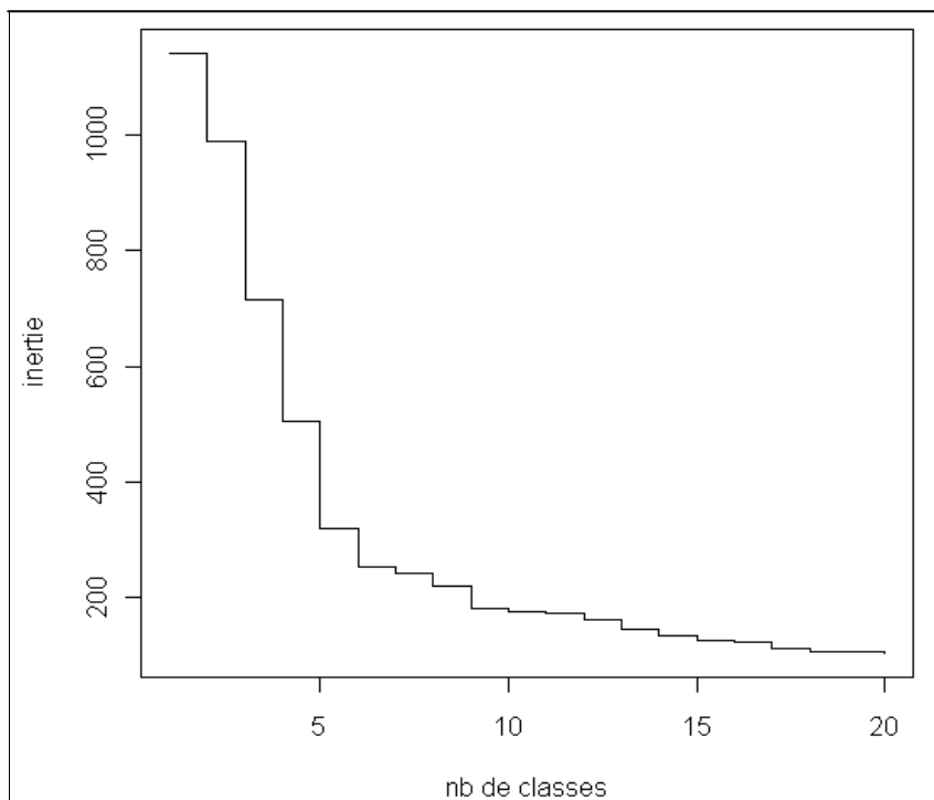
Figure 4b – Inertie de la partition selon le nombre de classes
