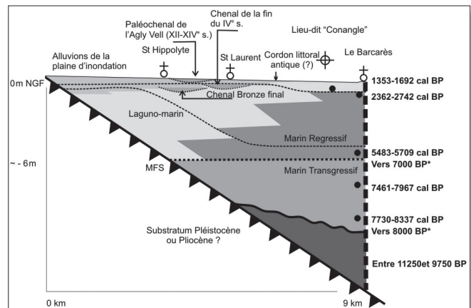
Fig. 1 - Reconstitution de la position des littoraux vers 10500, 8400 et 6000 ans BP et ses relations avec les formations Holocènes continentales en Roussillon – Schéma : Carozza, 2011
