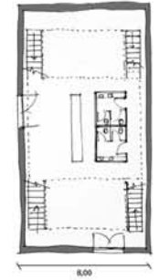
RÉZ-DE-CHAUSSÉE
