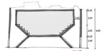
COUPE
