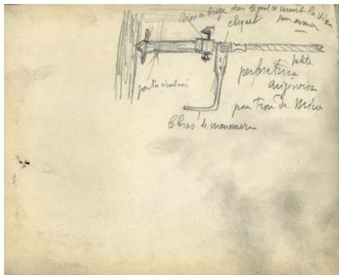
Dessin 7 : [ Perforatrice anzinoise pour trou de mine ] Mine de plomb et fusain l. 26,5 x H. 21,2 cm Inscription de la main de l'artiste : « petite perforatrice anzinoise pour trou de mine ; écrou en bronze dans lequel on met la visse [sic] pour armer ; cliquet ; partie circulaire ; bras de manoeuvre ».
