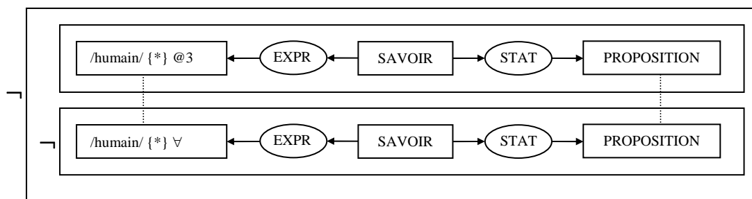
Figure 11 : molécule lexicalisée par ce que trois savent, tous le savent
