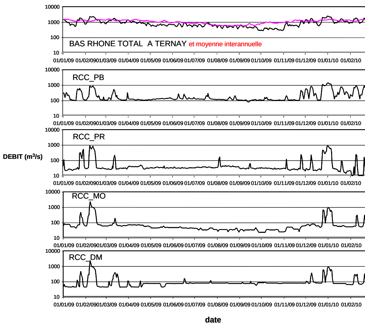
Figure 2.1.2 : Débit 2009 du Rhône total à Ternay, et dans les vieux Rhône du bas Rhône
