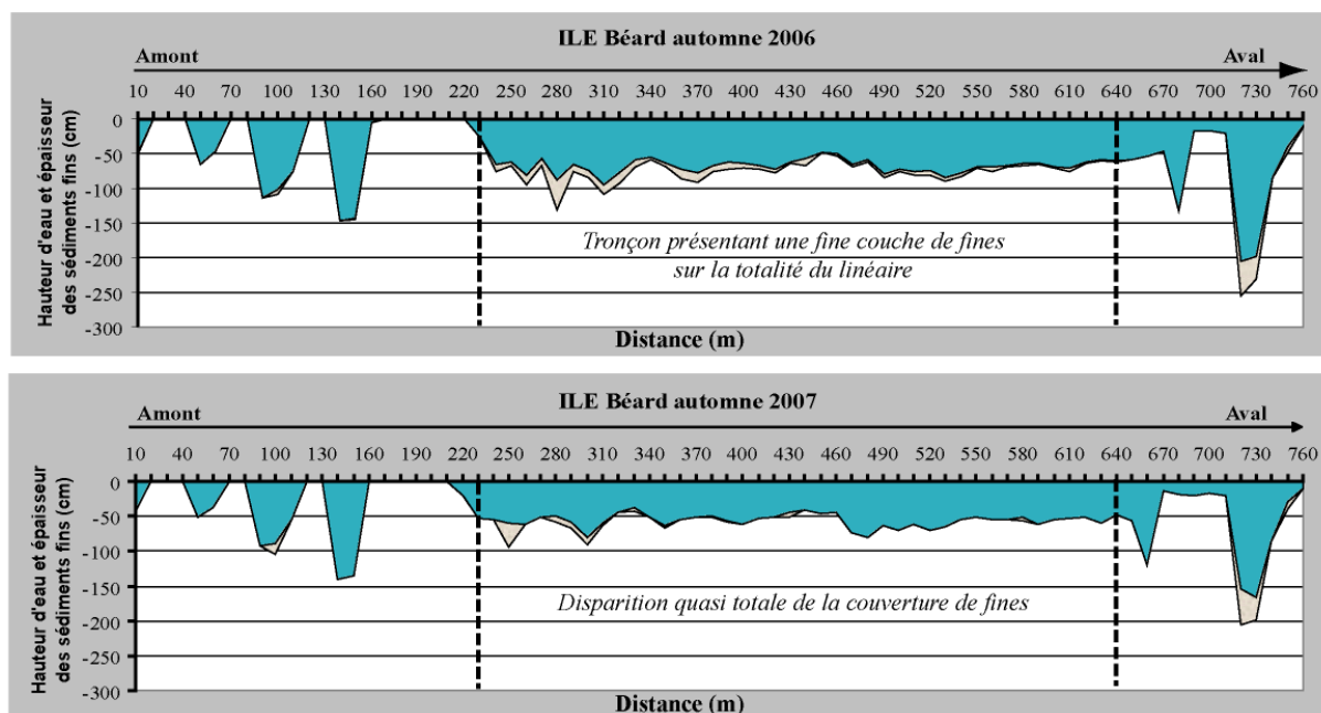
Figure 3.4.3 : Mise en évidence d'une phase où les processus de décavage dominant sur la sédimentation. L'exemple de BEA entre octobre 2006 et Octobre 2007.
