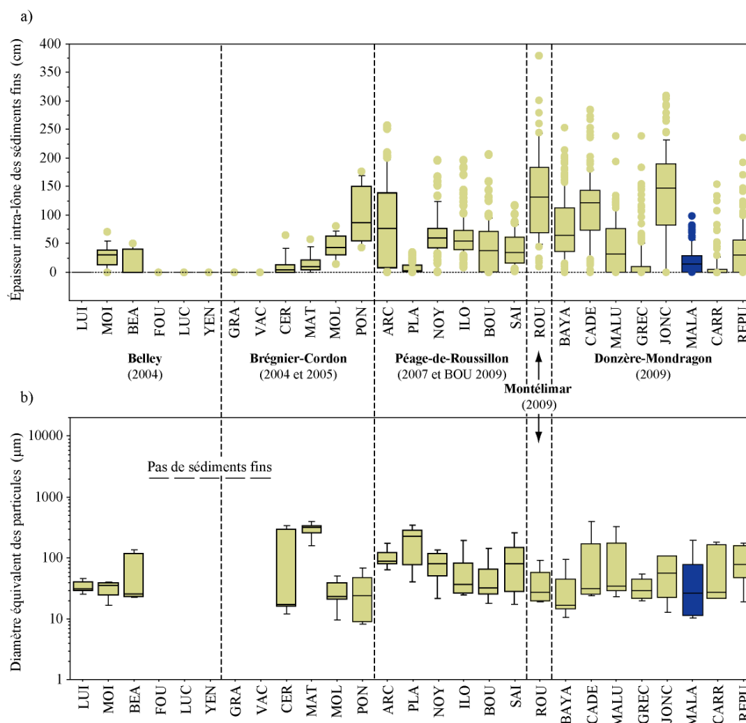
Figure 2.4.1 : Analyse synchronique de l'évolution de l'épaisseur sédimentaire (a) et du D50 moyen (b) des îlots non réhabilités sur le continuum rhodanien. (La îlot de Malatras donne un aperçu de la réponse d'un système restauré sur le Rhône moyen – taux de sédimentation = 5,1 cm/an). En ce qui concerne l'épaisseur sédimentaire, le nombre d'échantillons considéré pour chaque îlot non-réhabilité est indiqué sur les graphiques de l'annexe 4.4.1. Les données granulométriques reposent sur une base de cinq échantillons par îlot).
