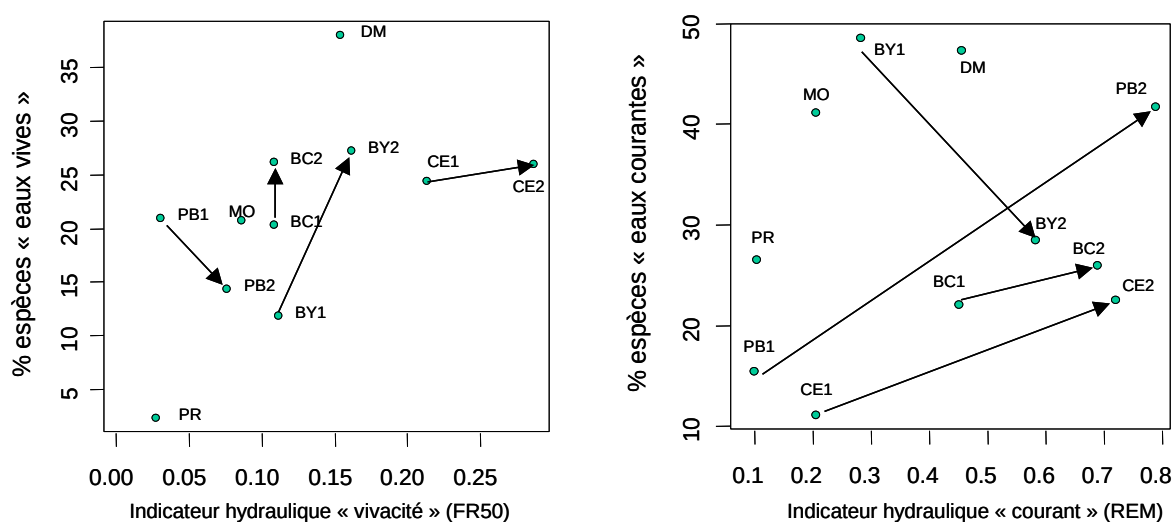
Figure 2.2.3 : Evolution des indicateurs hydrauliques et indicateurs 'poissons' associés reflétant l'abondance relative des espèces d'eau courante (à droite) et d'eau vive (à gauche).
