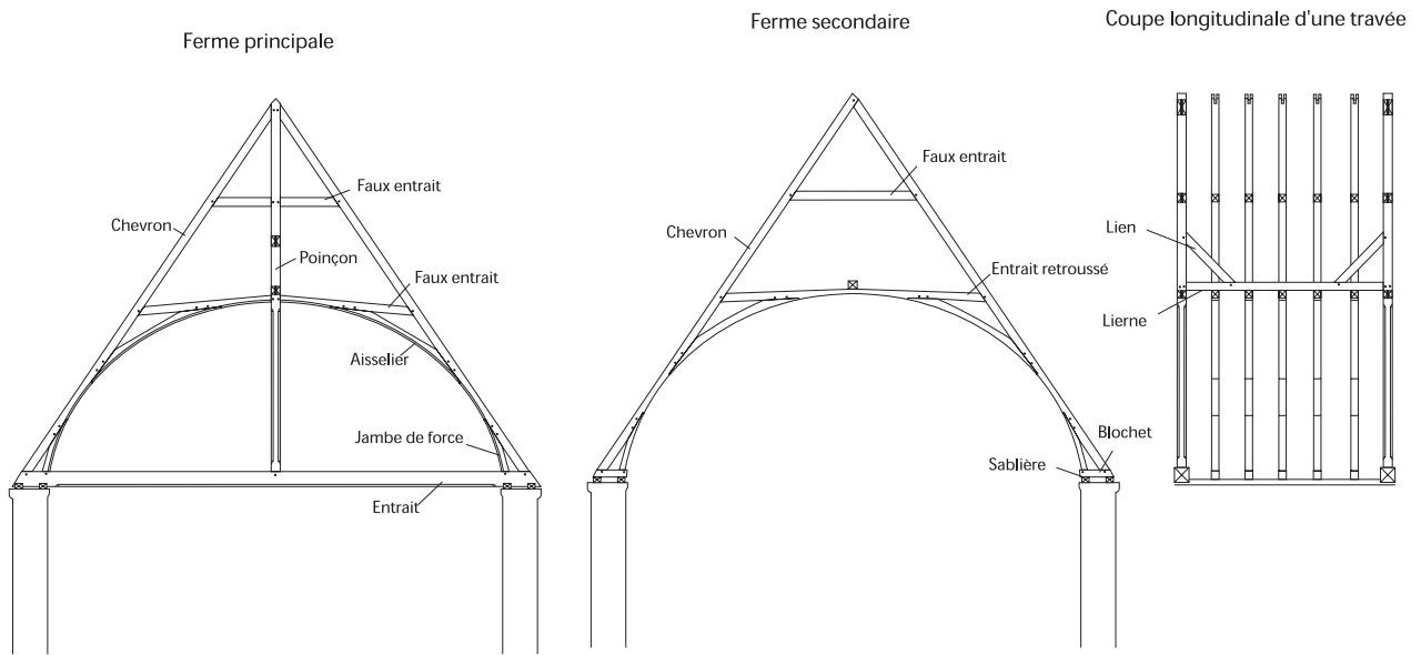
Fig. 32 : Abbaye de Royaumont. Comble du dortoir des convers. Ferme de la charpente voûtée du XIII e s. réemployée au XIX e s.
