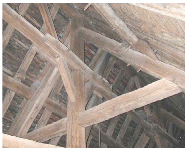
Fig. 47 : Église Saint-Didier de Villiers-le-Bel. Moises des sous-faîtières dans la charpente du chœur, XVI e s.
