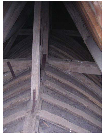
Ferme et cerces de la nef
