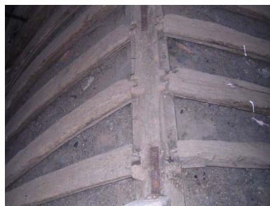
Assemblages des cerces dans la sous-faîtière
