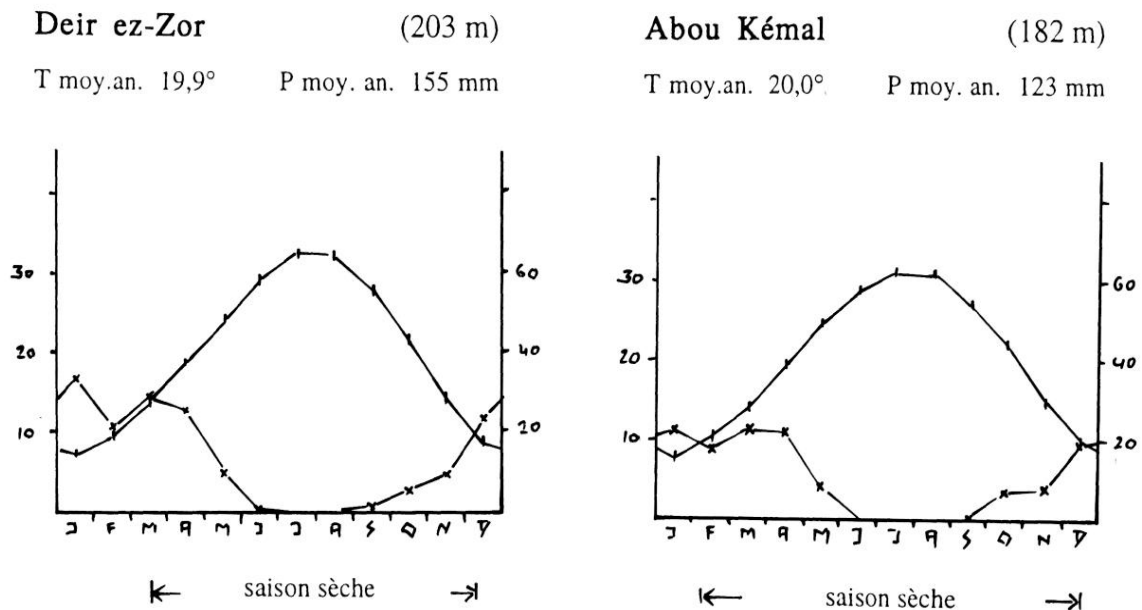
Fig. 1 : Diagrammes ombrothermiques pour les stations climatiques de Deir ez-Zor et Abou Kémal (d'après M. Alex, 1985).
