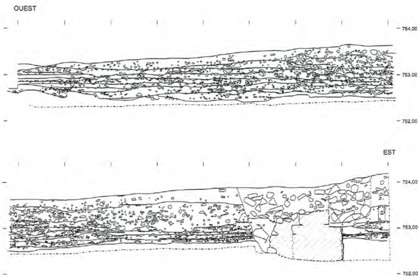
Fig. II.3.1 : La grande rue de la Pâturerie du Couvent : relevé stratigraphique au sud du bassin naviforme.
