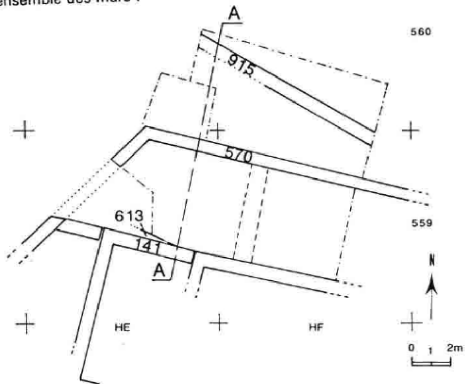
Plan d'ensemble des murs .
