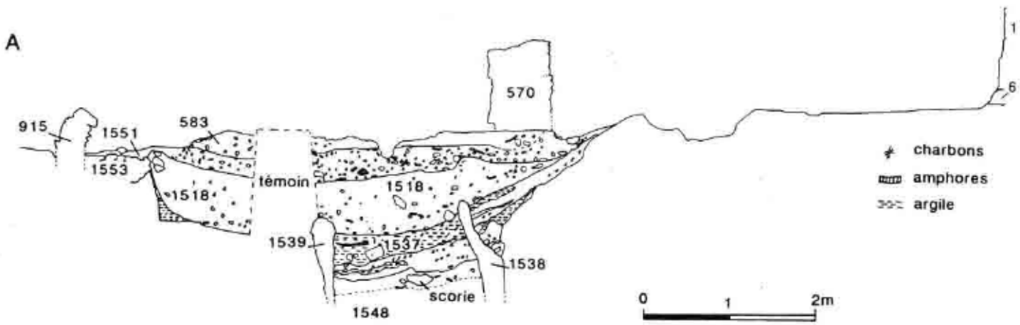
Coupe de la cave à armature en bois.
