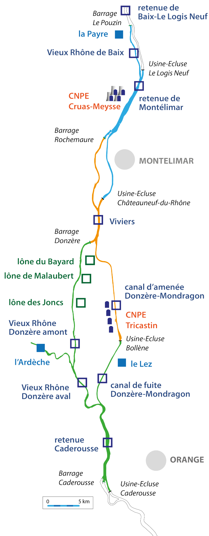
Figure 9.1 - Schéma des aménagements hydro-électriques du Bas Rhône Médian. Localisation et dénomination des stations d'échantillonnage des poissons
