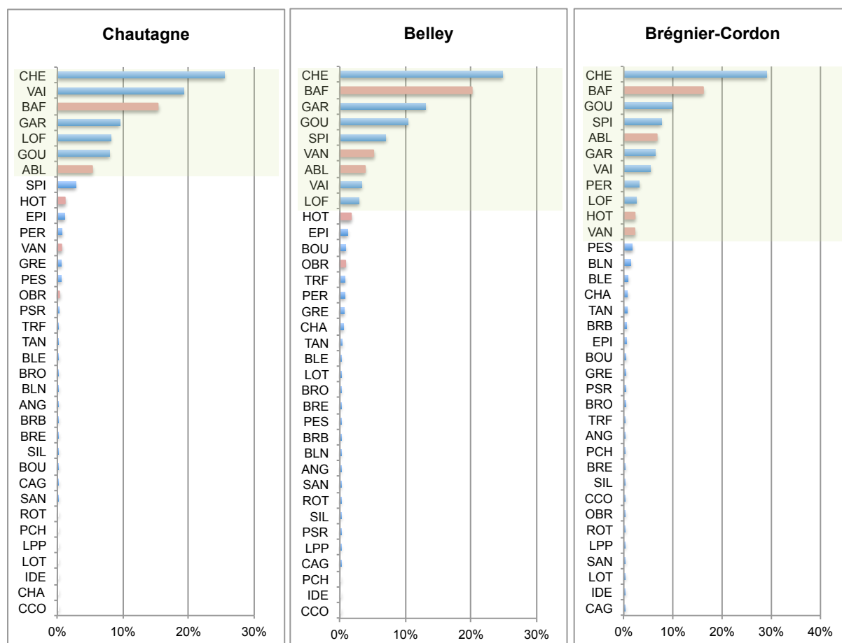
Figure 4.1 - Abondances relatives des différentes espèces échantillonnées après augmentation des débits réservés dans les trois vieux-Rhône de Chautagne, Belley et Brégner-Cordon. Les valeurs correspondant aux espèces « d'eau courante » sont indiquées en rouge. Le cadre vert regroupe les espèces dont le cumul des abondances relatives correspond à 90% des effectifs échantillonnés.
