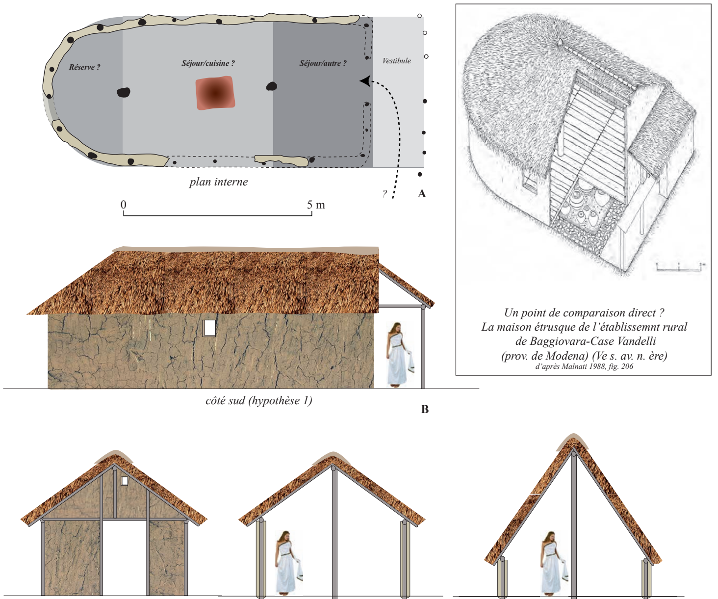
■ Fig. 32 : Proposition de restitution de l'UNF145.
