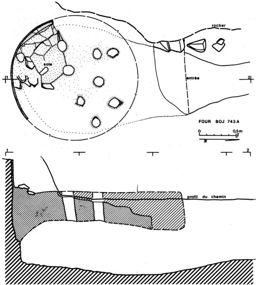
Pl. III - Plan et coupe axiale du four BOJ 743 A
