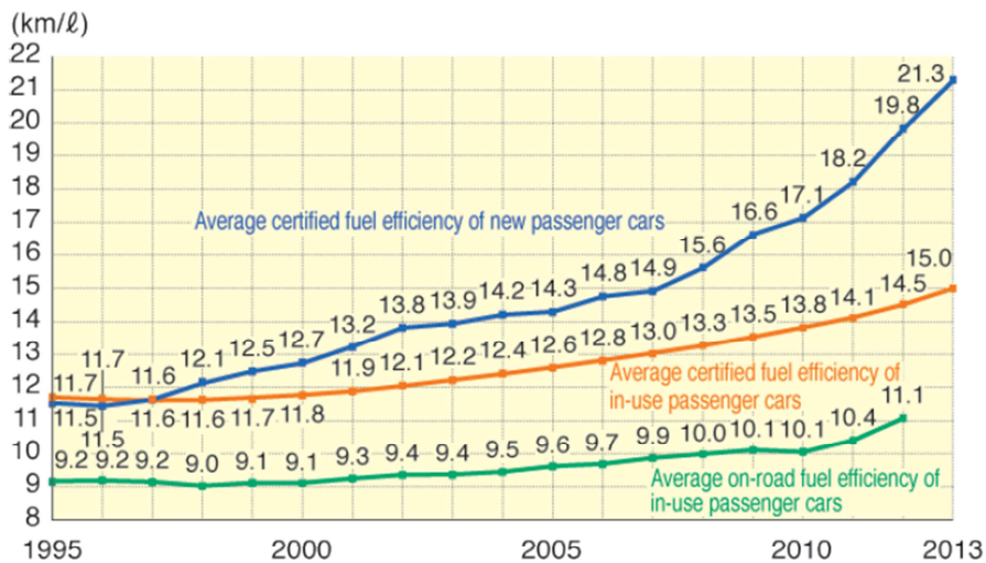
Figure 3.16 : Amélioration de l'efficacité énergétique des véhicules au Japon
