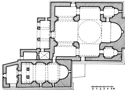
Pl. 37a - Sapara (fin du XIII e - début du XIV e s.). Plan
