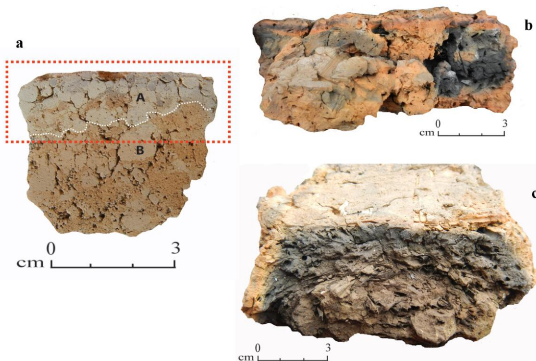
Fig. 15. Esempi di caratteri strutturali grumosi: (a) Solarolo-via Ordiere (RA), scavi UNIBO, elemento con struttura grumosa composta da aggregati massivi scarsamente coalescenti (A), impostata su un livello caratterizzato da un assemblaggio eterogeneo di aggregati massivi e sacche sabbiose (B); (b-c) Marais Vernier (dipartimento dell'Eure, Haute Normandie, Francia), campioni provenienti da edificio attuale distrutto da incendio: b) struttura grumosa composta da aggregati con grado di coalescenza variabile; c) struttura grumosa con aggregati da fortemente a mediamente coalescenti, localizzate aree massive.
