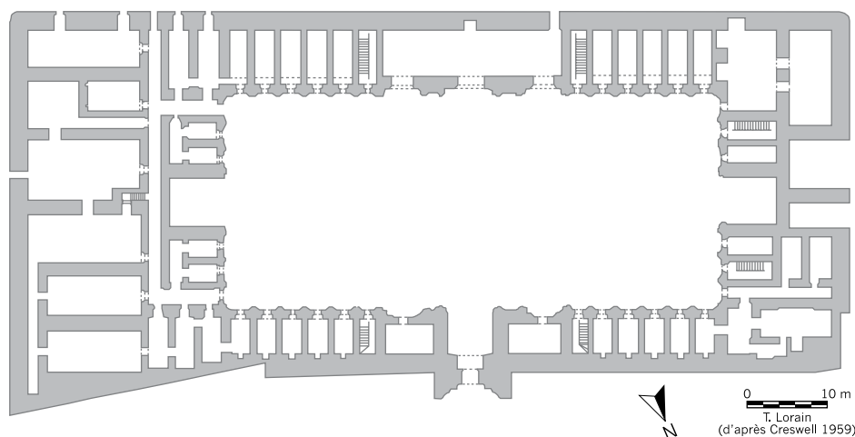
Plan de la madrasa Mustansiriyya de Bagdad, 1233.
