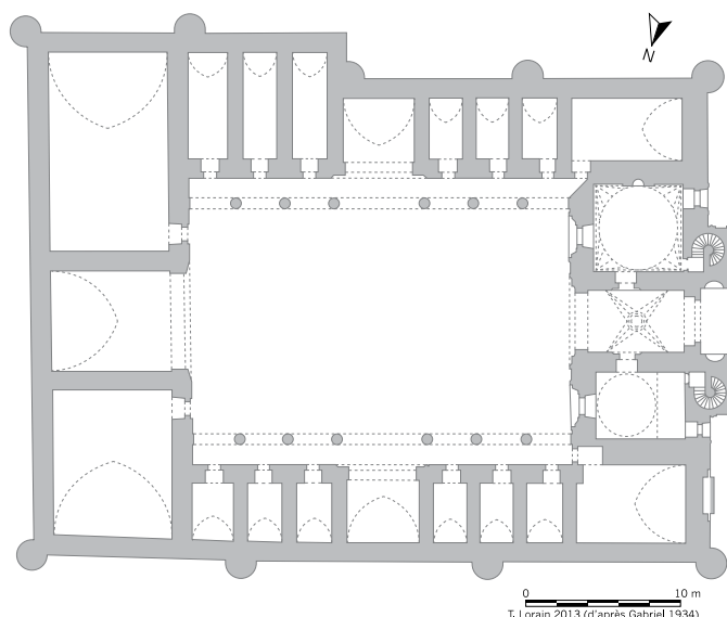
Plan de la Gök medrese de Sivas, fondée en 1271.
