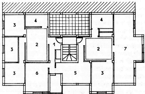
Ill. 4 Plans d'origine de la même maison
