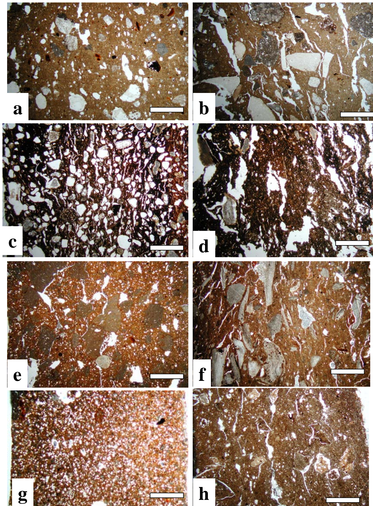
Figure 4 Illustration des différents pétrofaciès rencontrés dans les assemblages des céramiques chalcolithiques du Levant Sud. Figures 4a & 4b. Assemblage homogène illustré par Tell Sabarta (Pella). 4a : pôle fin montrant quelques inclusions sableuses subarrondies incorporées à une argile calcitique fine très bien préparée ; 4b : pôle grossier montrant une proportion élevée de sables grossiers anguleux incorporée à une argile calcitique fine assez bien préparée. Dans les deux cas, la masse fine et la fraction grossière proviennent des formations superficielles dérivées des marnes éocènes présentes sur tous les environs du site. Les
