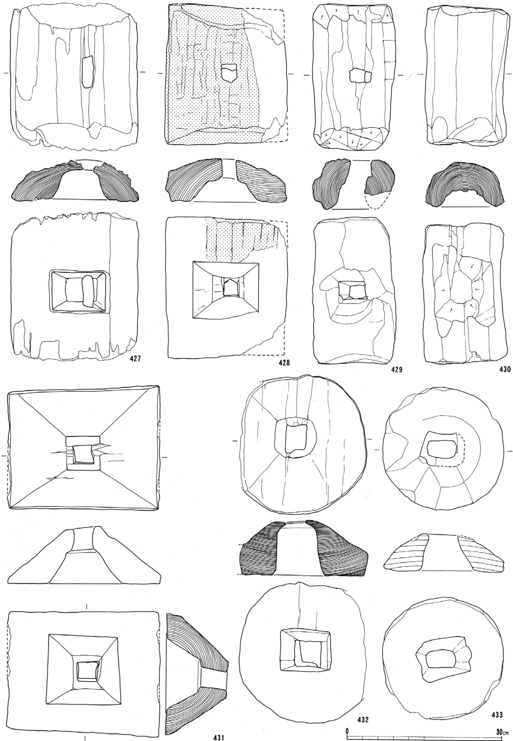
第32図 タタリ(427~433)
