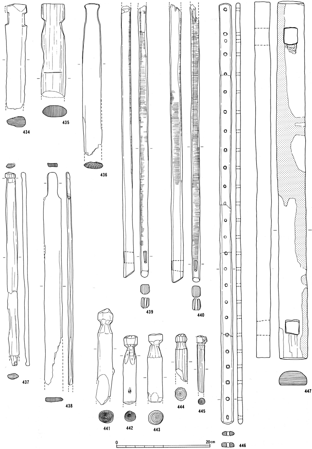
第33図 織機(434~447)
