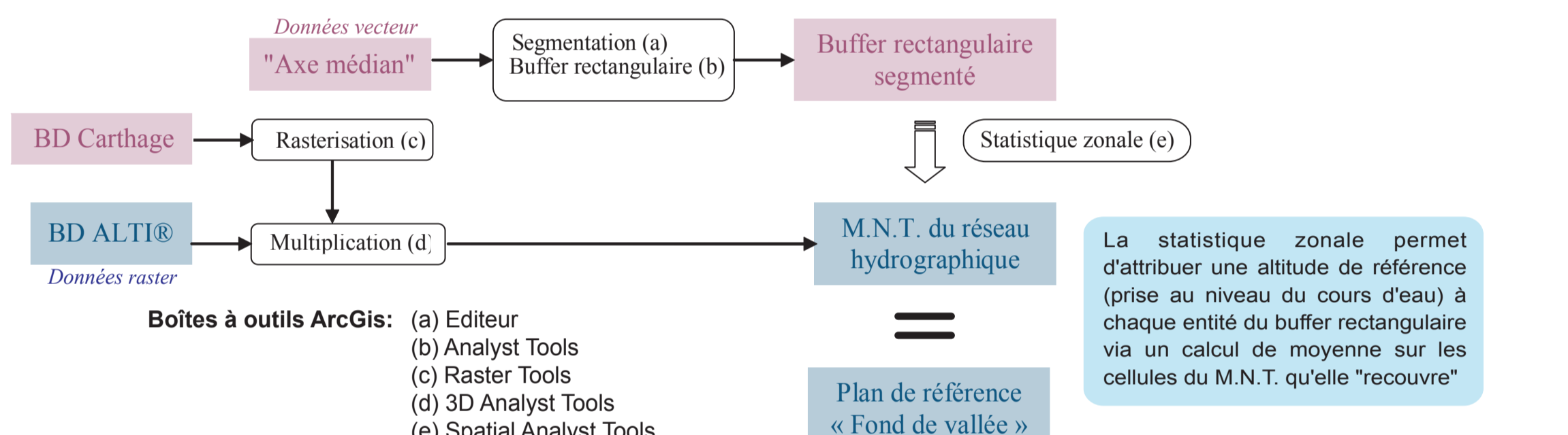
Figure 5: Test du critère de pente (méthode 1) pour déterminer les fonds de vallée
