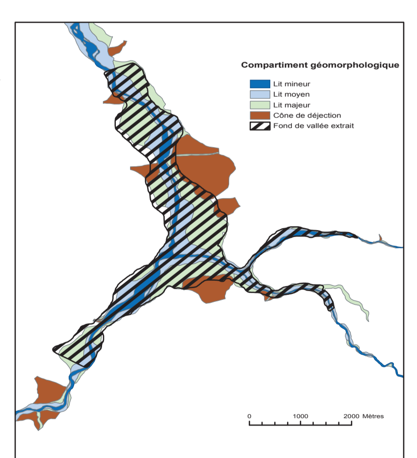
Figure 9 : Superposition de la cartographie hydrogéomorphologique à la plaine alluviale extraite
