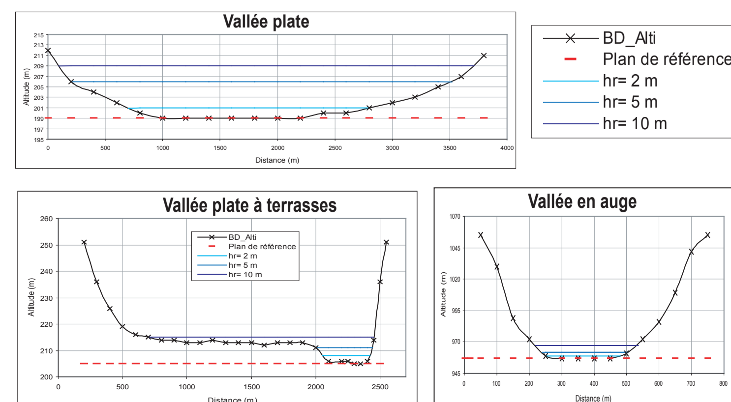
Figure 10 : Sensibilité de la largeur de plaine au seuil de hauteur retenu pour différents profils de vallée
