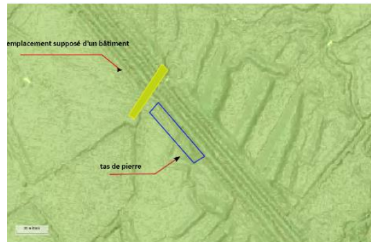
Figure 11 : Carte LIDAR
