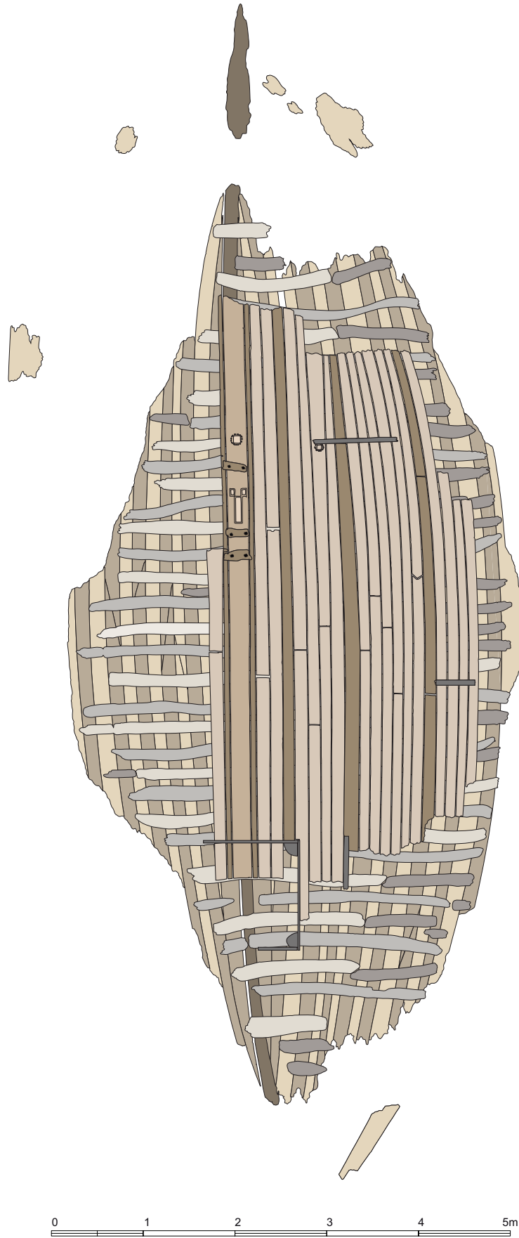
Fig. 1 : Planimétrie des vestiges (P. Poveda d'après Santamaria 1995).
