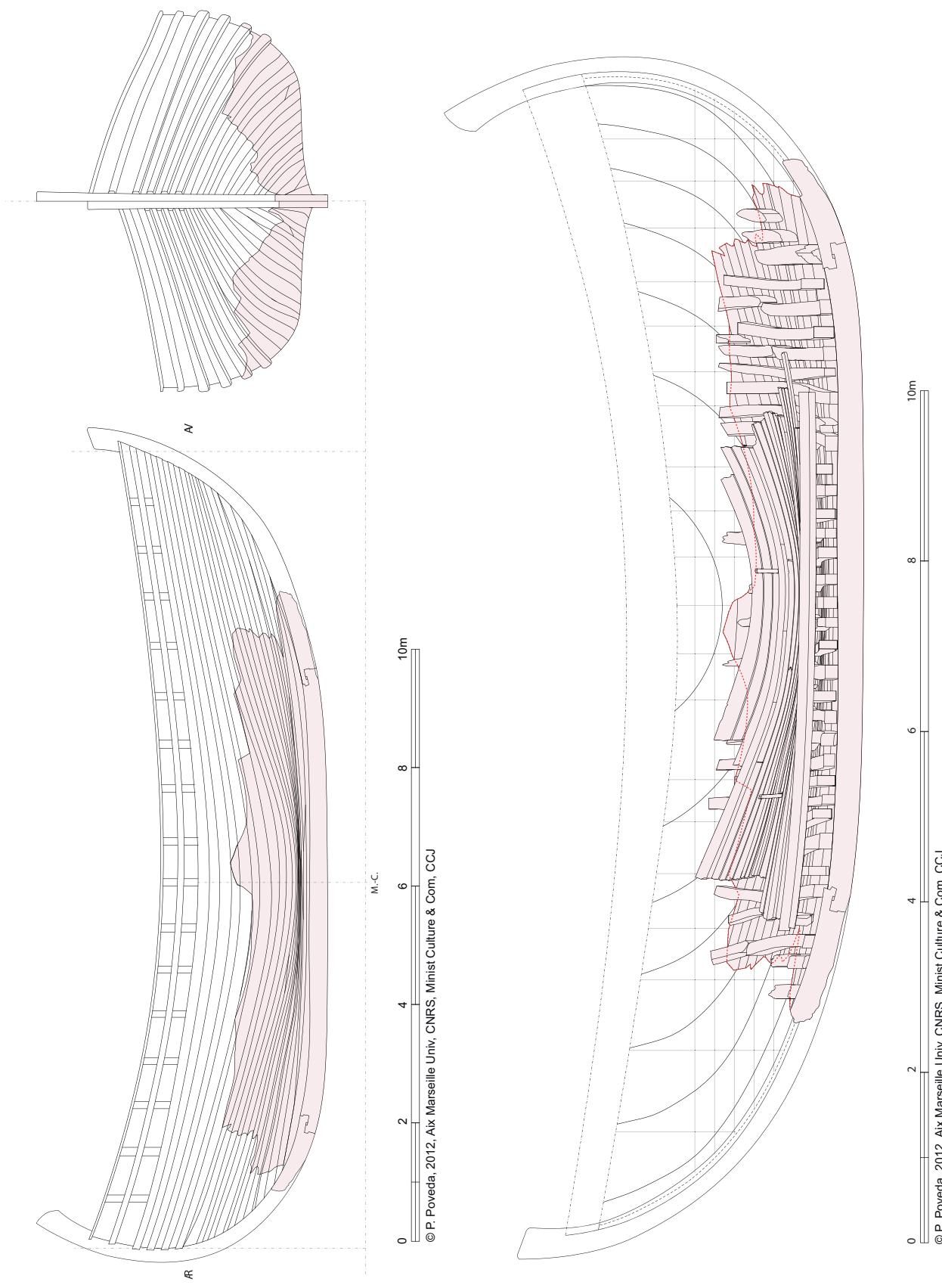
Fig. 5 : Plan de coque et vue longitudinale des vestiges remis en place au sein du plan de formes de restitution (P. Poveda).
