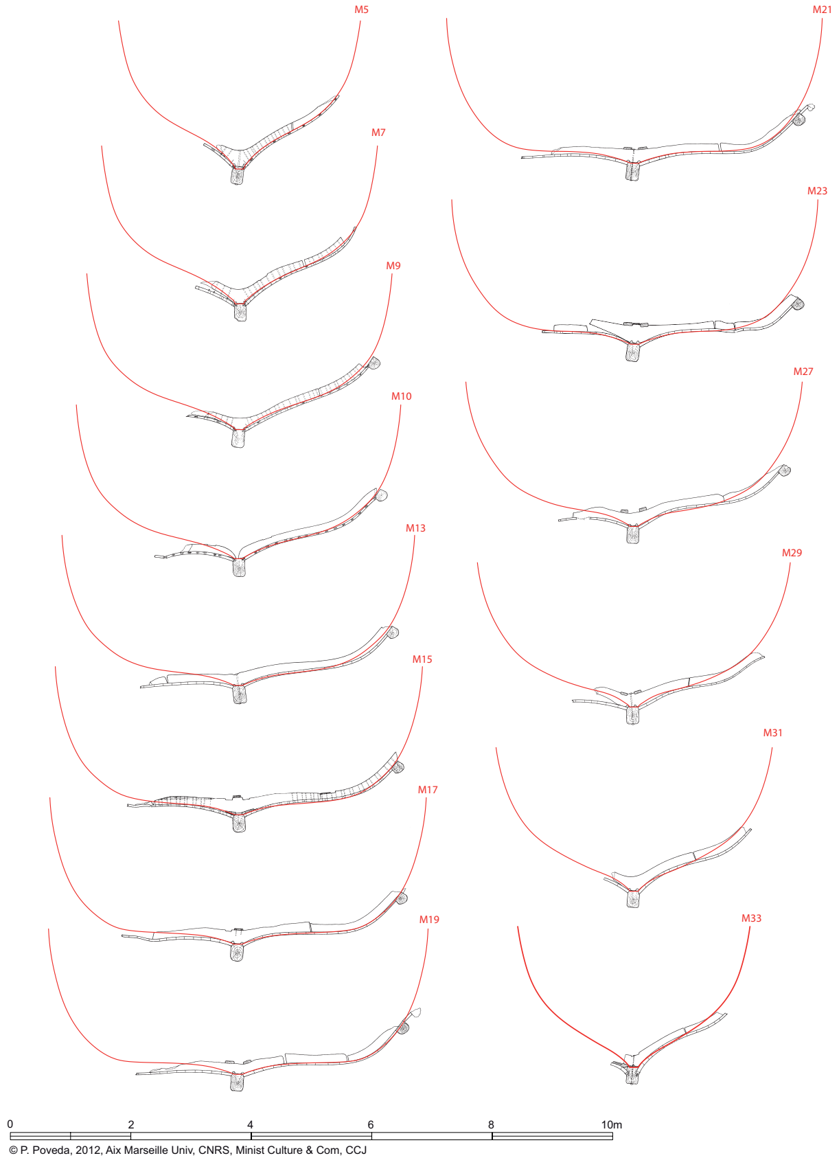
Fig. 2: Vue de la remise en place des coupes transversales des vestiges sur les coupes du plan de formes de restitution (P. Poveda).
