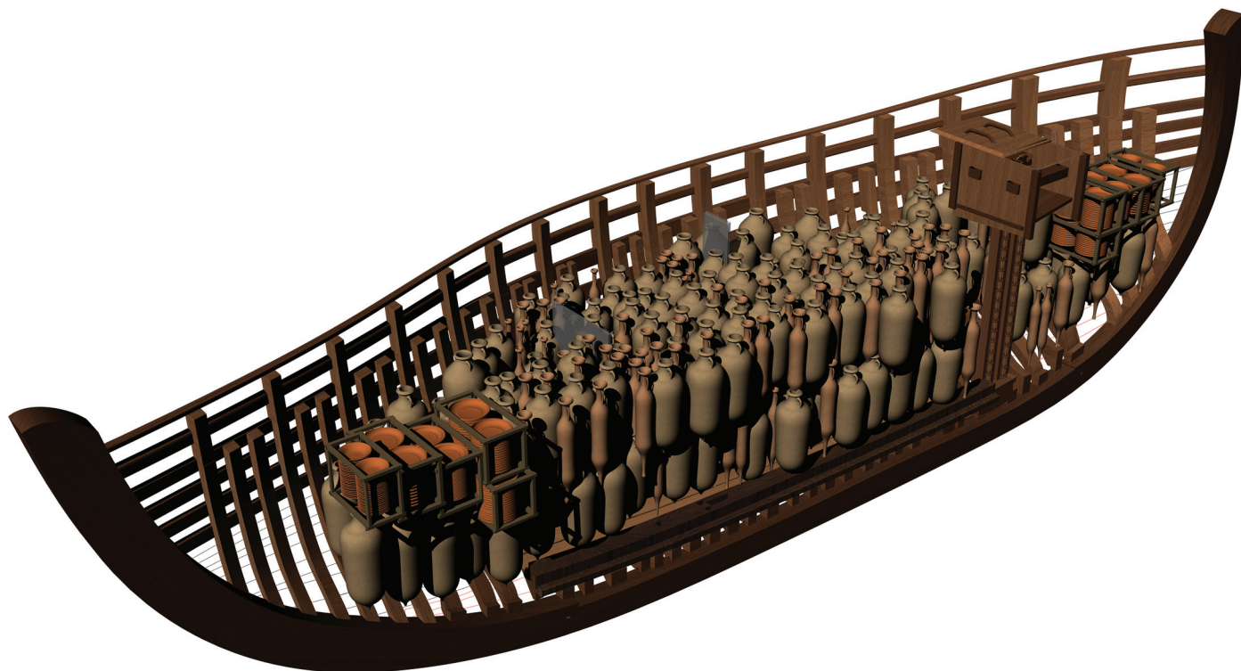
Fig. 7 : Vue de trois-quarts du modèle 3D de restitution du flanc tribord et de la cargaison (P. Poveda, CCJ/AMU/CNRS).
