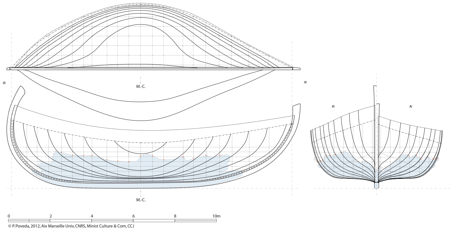
Fig. 4: Plan de formes de la deuxième hypothèse de restitution (P. Poveda).
