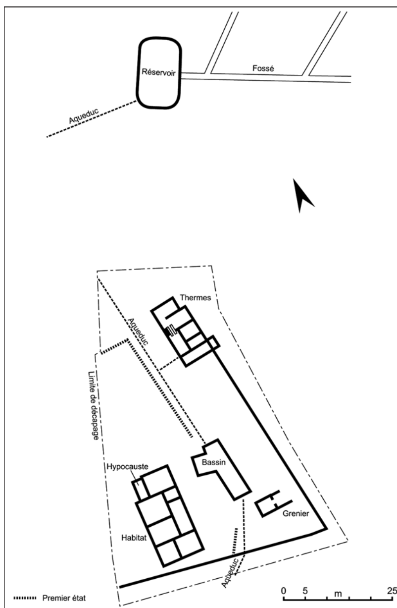
11. Plan de la villa de Puy Gilbert Sud à Prondines (d'après Rebiscol 2005)
