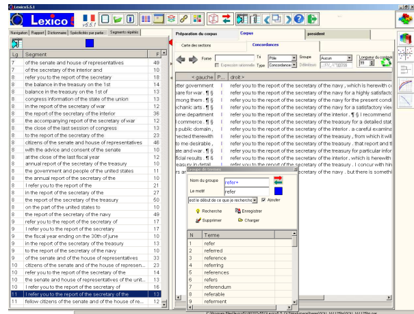
Figure 5.b : Lexico 5.5.1, Segments Répétés et Tgen Corpus STATE OF THE UNION. Concordance d'un long segment répété et construction d'un groupe de termes commençant par « refer »
