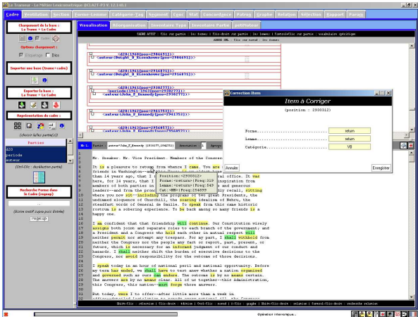
Figure 6.a : Trameur 12.148.1, Visualisation du Cadre, Coloration, Correction d’un item Corpus STATE OF THE UNION. On a choisi de surligner les verbes en jaune et les modaux en vert. On repère une occurrence du verbe
