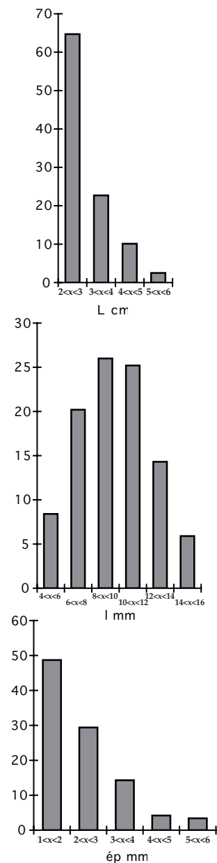
Fig. 23 - Dimensions des produits laminaires.
