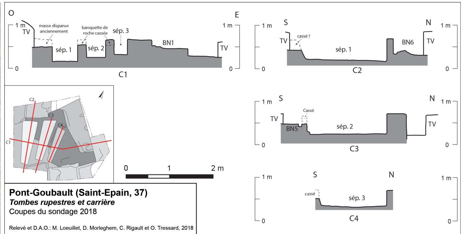
Fig. 21 - Relevés des sections des tombes rupestres
