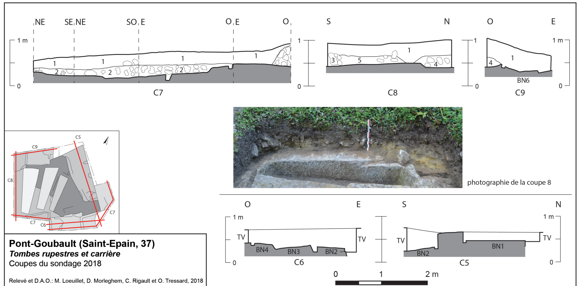
Fig. 22 - Relevés des coupes stratigraphiques du sondage 2018
