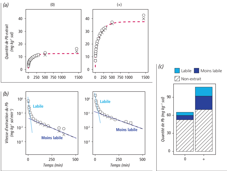
Figure 4. Extraction cinétique d'un horizon de surface pour un sol du secteur non contaminé (0) et un sol du secteur moyennement contaminé (+). (a) Quantité de plomb extrait en fonction du temps, (b) vitesse d'extraction du plomb en fonction du temps pour les deux secteurs étudiés, et (c) quantité de plomb non-extrait, « moins labile » et « labile » dans l'horizon analysé.
