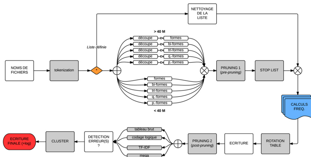
Fig. 4. Schéma global du programme Text-to-CSV, développé dans le cadre de nos recherches et largement employé lors des analyses. Le répertoire de fichiers passe par différents traitements, visant à les nettoyer ( tokenization ), puis à générer une liste de mots ou groupes de mots (appelés n-grams ; liste potentiellement fournie par l'utilisateur) dont les fréquences sont ensuite calculées pour chaque sous-corpus/fichier. Différents traitements peuvent enfin être appliqués (rotation de la table obtenue, élagage des résultats et applications de coefficients), avant une vérification finale.
