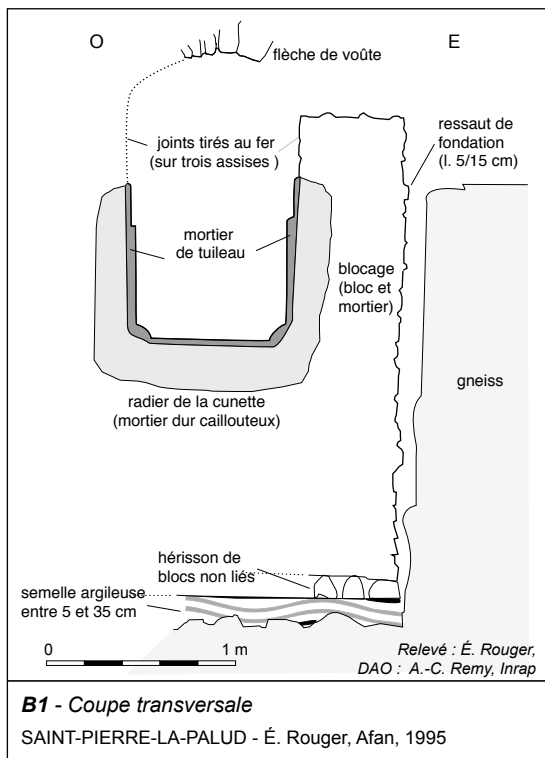
Fig. 17. Les fondations, passages enterrés, aqueduc de la Brévenne.
