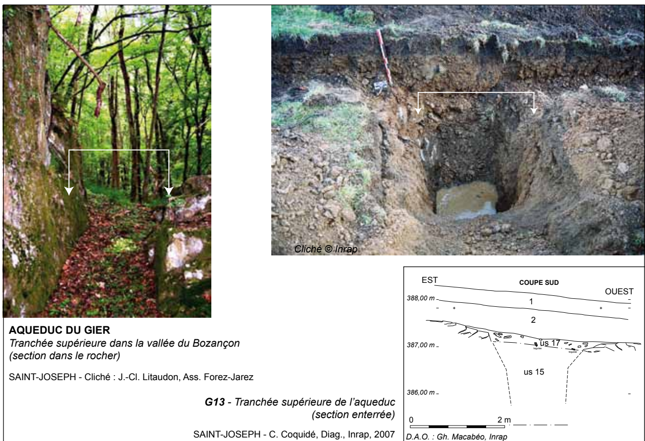
Fig. 36. La tranchée supérieure de l'aqueduc du Gier.
