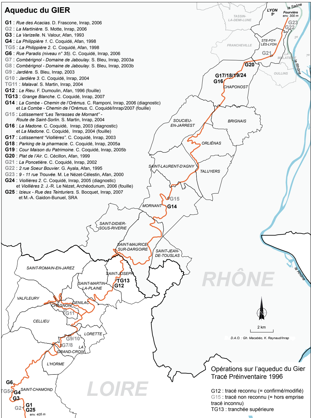
Fig. 5. Tracé et opérations sur l'aqueduc du Gier.
