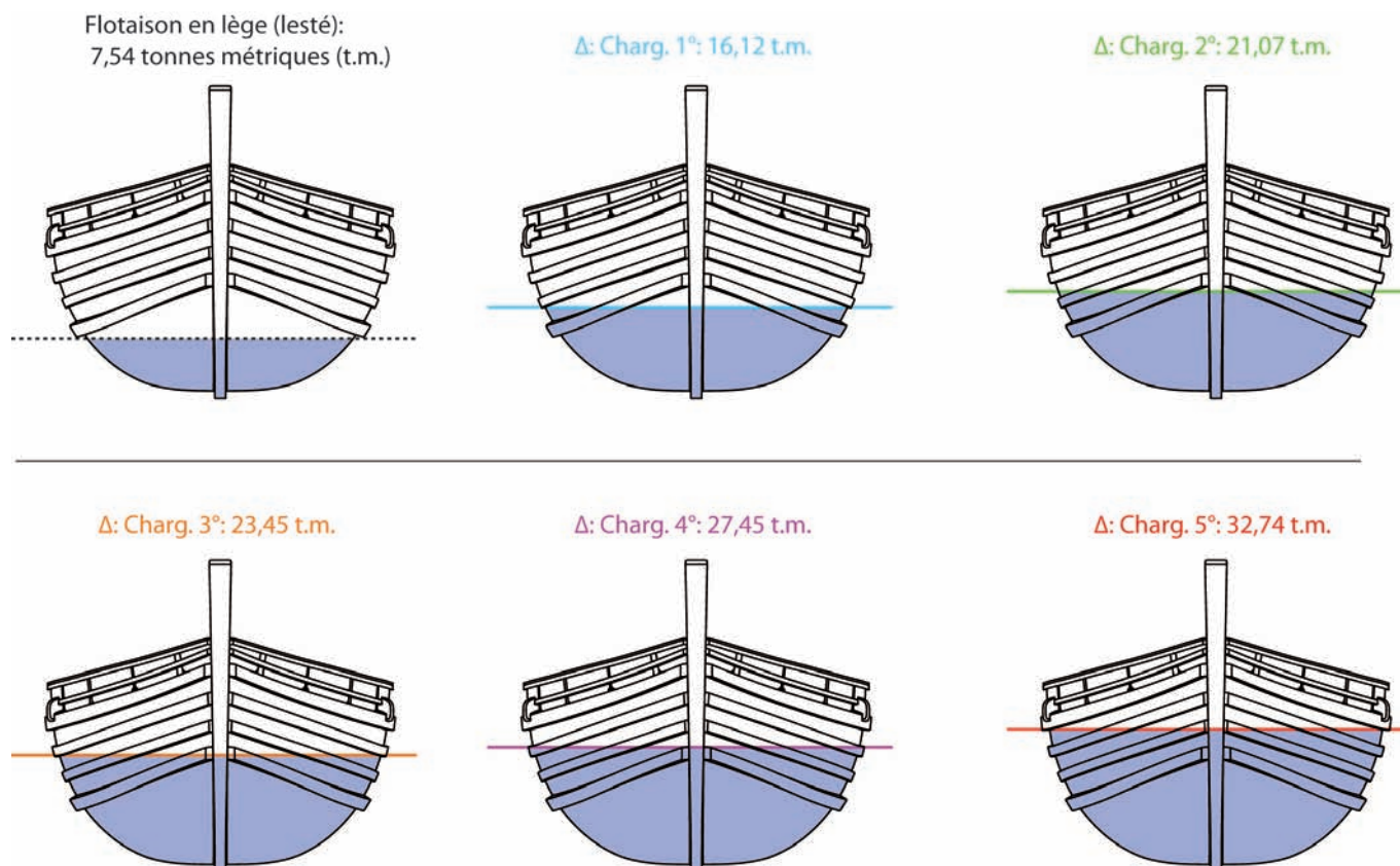
Fig. 44 : Représentation des différentes lignes de flotaison au niveau du maître-couple en fonction des divers chargements (les différentes vues ne tiennent pas compte de l'inclinaison longitudinale, ou assiette, résultant de chaque chargement) (dessin P. Poveda).
