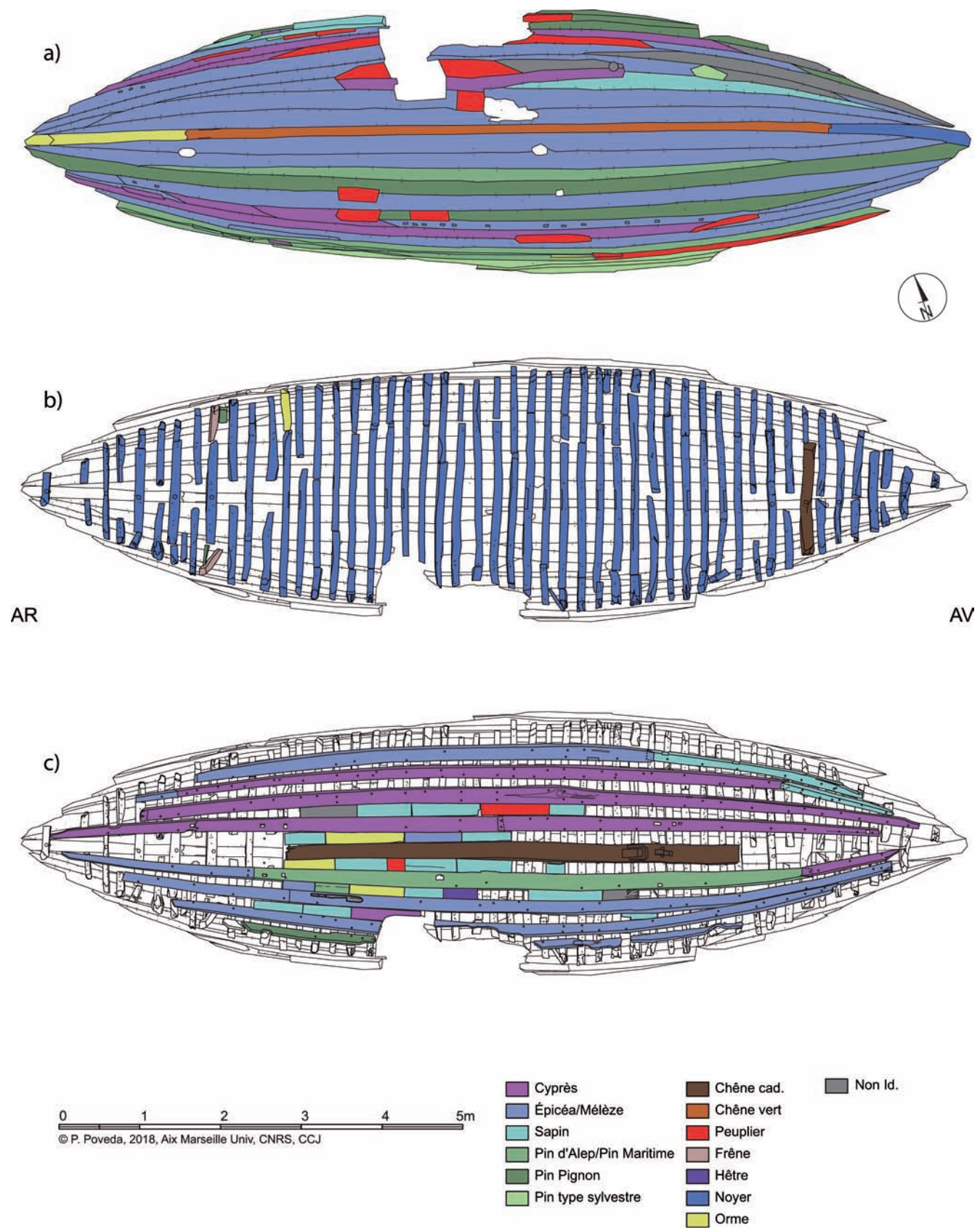
Fig. 38: Distribution des essences de bois dans les vestiges conservés: a. charpente axiale et bordé face extérieure; b. membrure; c. charpente longitudinale interne (relevé Tecno In. e et Calcagno Architetti Associati, DAO P. Poveda).
