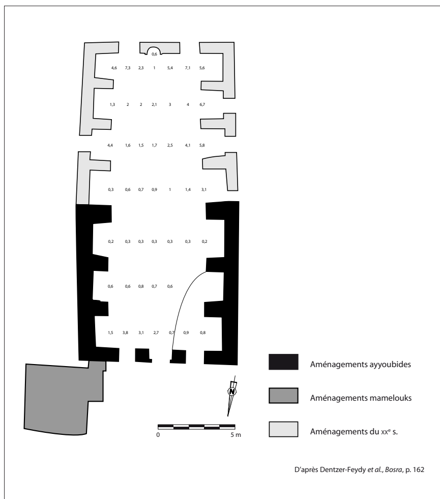
Fig. 1. Mosquée de Fāṭima : étapes de construction et éclairage exprimé en facteur de lumière du jour.
