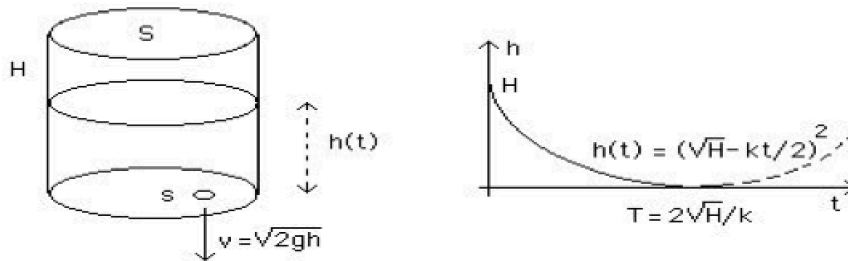
Figure 12 – Si un vase se vide par un petit trou...
