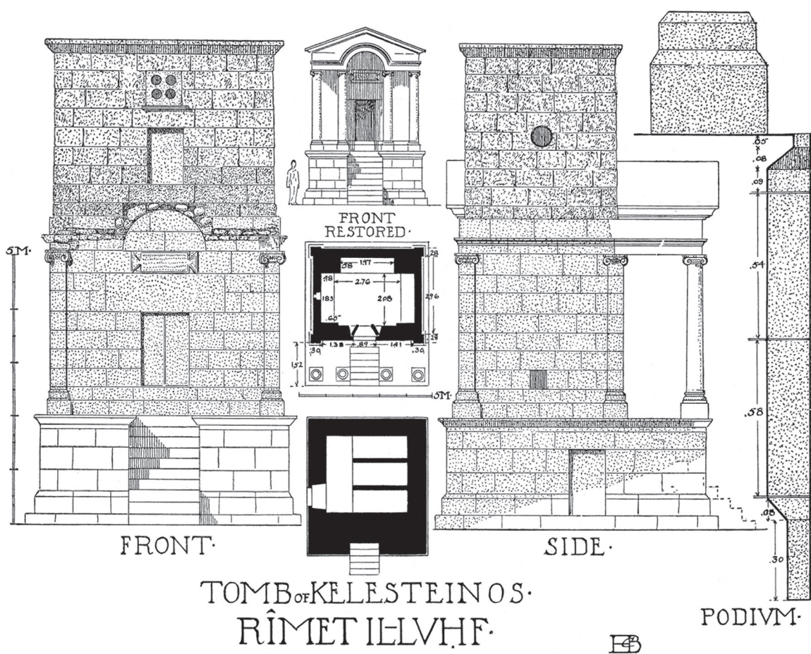
Figure 4 : Tombeau de Célestinus à Rimat al-Luhf (relevés en plan et en élévation, proposition de restitution d'après BUTLER 1919, p. 413, fig. 354)
