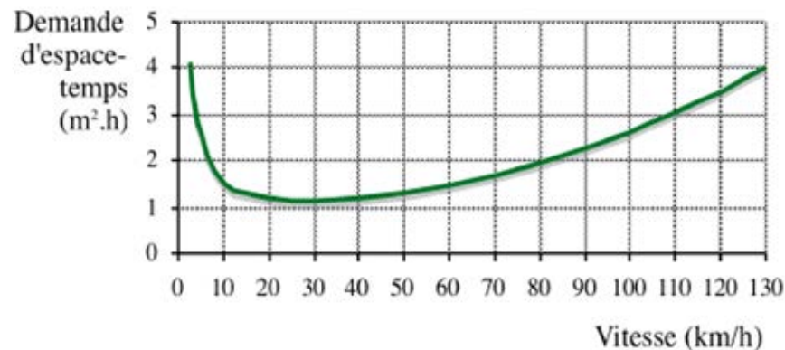
Figure 1 : consommation d'espace-temps d'une automobile en fonction de sa vitesse
