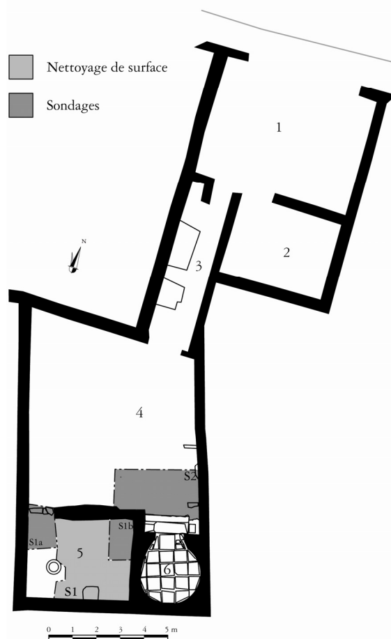
Fig. 4. Plan, nomenclature et localisations des opérations effectuées durant la campagne 2008 dans la boulangerie VII 12, 13 (relevé: F. Fouriaux – V. Lallet, C. Loiseau – S. Zanella).
