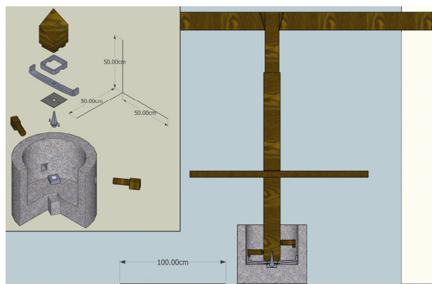
Fig. 12. Restitution du pétrin de la maison des «Chastes amants» (IX 12, 6); éclaté isométrique et coupe (échelle 1/50; dessins N. Monteix).
